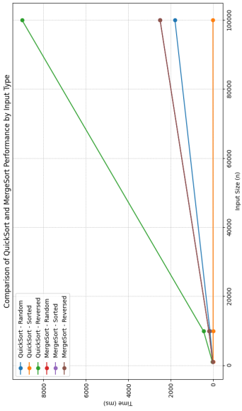
Figur 1: Exekveringstid för de två sorteringsalgoritmerna QuickSort och MergeSort i Scala. För båda algoritmerna plottas tre olika indatatyper separat: Slumpmässig, sorterat och omvänt sorterad indata. (Linjär skala)
