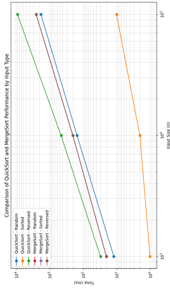
Figur 2: Exekveringstid för de två sorteringsalgoritmerna QuickSort och MergeSort i Scala. För båda algoritmerna plottas tre olika indatatyper separat: Slumpmässig, sorterat och omvänt sorterad indata. (Logaritmisk skala)
