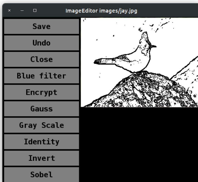
Figur 12.5: Bildredigeringsfönstret med alla filter implementerade. Ett konturförstärkande så kallat Sobel-filter är applicerat med tröskelvärde 150.
