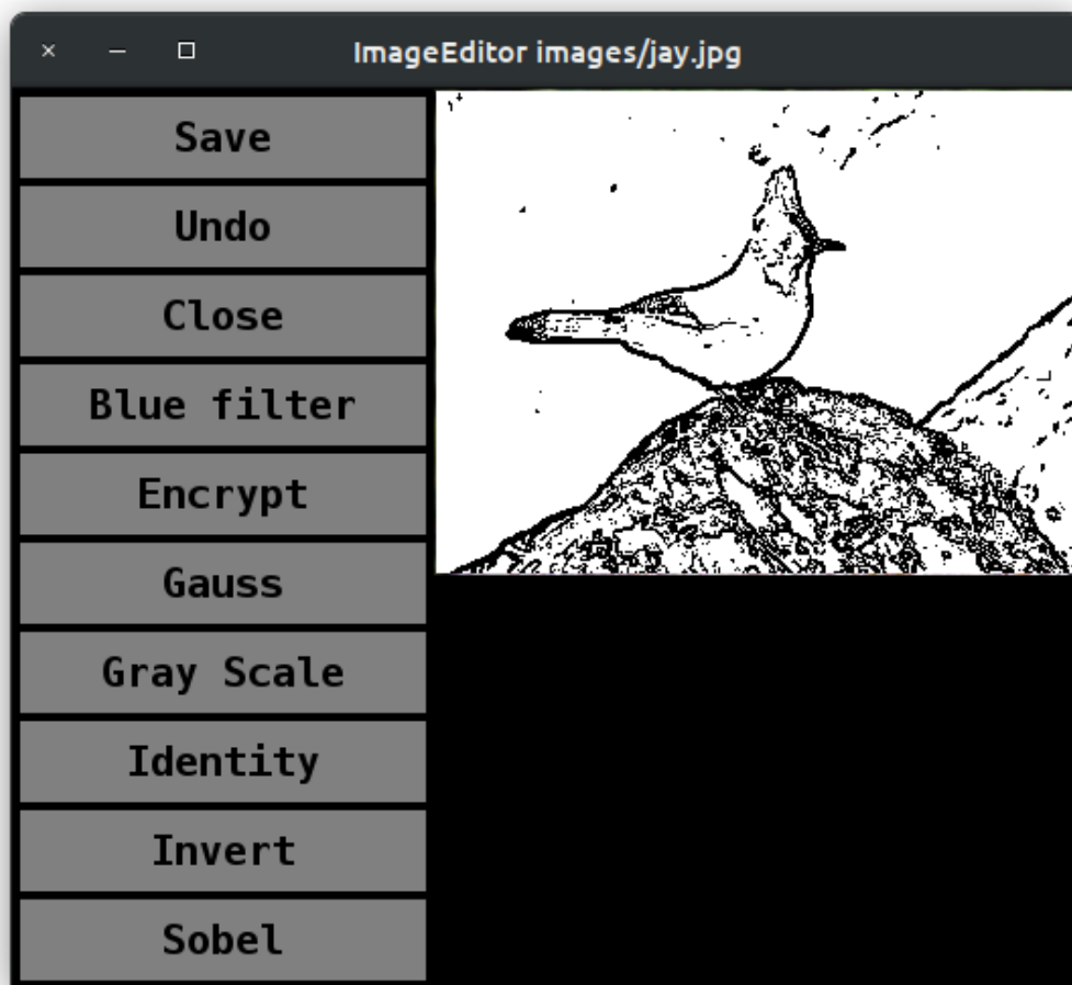
Figur 12.5: Bildredigeringsfönstret med alla filter implementerade. Ett kontruförstärkande så kallat Sobel-filter är applicerat med tröskelvärdet 150.
