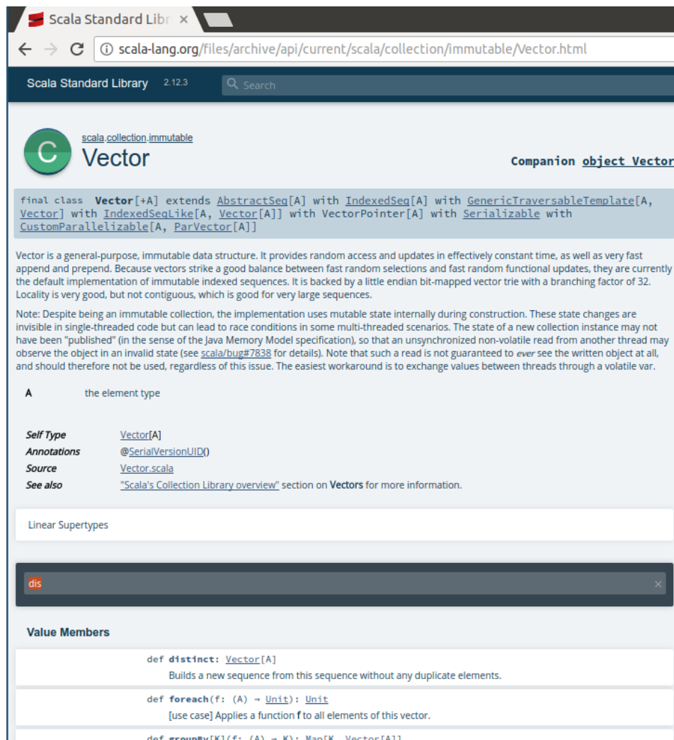
Figur E.4: En del av dokumentationen av klassen Vector
